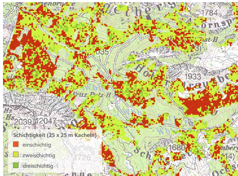
Abbildung 3: Darstellung der Bewertung der vertikalen Struktur (Schichtigkeit) in 25 x 25 m Kacheln, die mithilfe der Auswertung amtlicher Laserscanning-Daten ermittelt wurde. Einschichtige Kacheln sind gelb, zweischichtige rot und dreischichtige grün. Die Kacheln sind mit den großflächigen Lebensraumtypen verschnitten.
