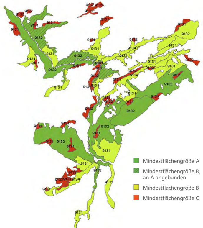
Abbildung 4: Analyse der Mindestgrößen und Verbundenheit von Teilflächen der großflächigen Lebensraumtypen am Beispiel des FFH-Gebietes Oberes Weißbachtal mit Lanzen-, Katzen- und Mittelbach.
